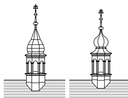
↑ Porovnání původní neodborné opravy sanktusníku s barokní a zároveň současnou
