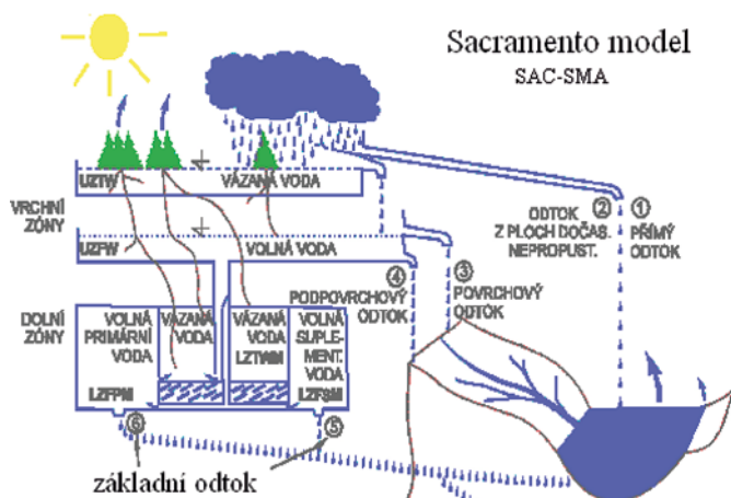
Obr. 3: Schema srážko-odtokového procesu pro počítačové simulace
