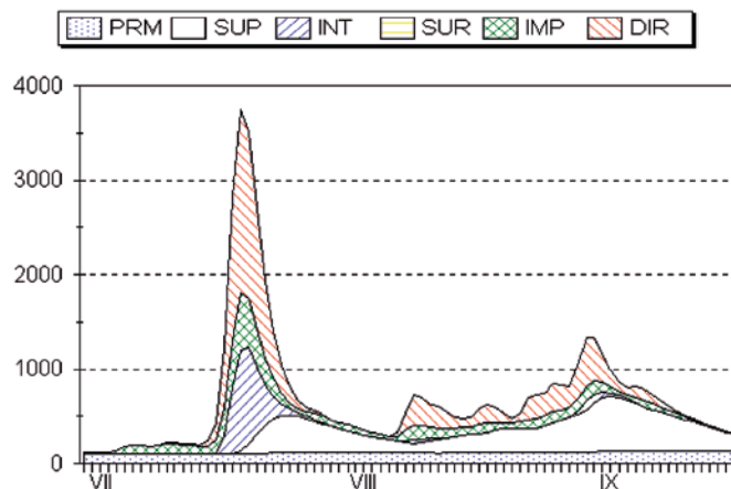
Obr. 4: Povodeň Labe-Děčín v roce 1954 sestávající z více složek simulovaných odtoků modelem Sac-Sma (pozn.: případ situace naplnění dobudované nádrže Slapy na Vltavě)
