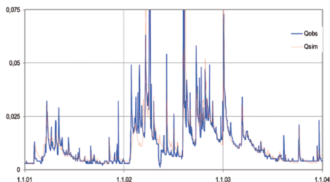
Obr. 5: Relativně dlouhé odtokové epizody indikují podpovrchový odtok v šumavském experimentálním povodí Liz (pozn.: roční období s jarním táním a extrémní povodní r. 2002 a suchým obdobím r. 2003)
