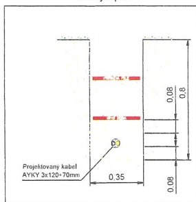
Rez výkopem
