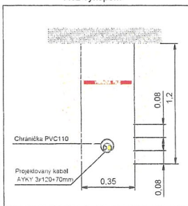
Rez výkopem
